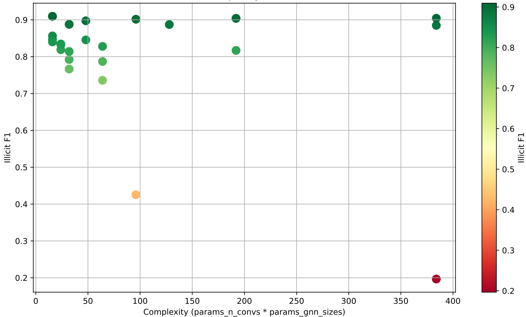
Illicit F1 vs Complexity for AMLSim 1/5
